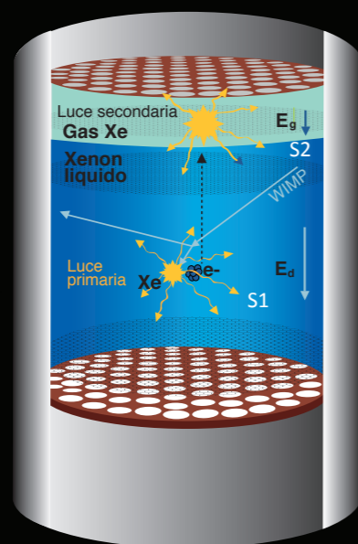
Rappresentazione schematica del rivelatore XENONnT
